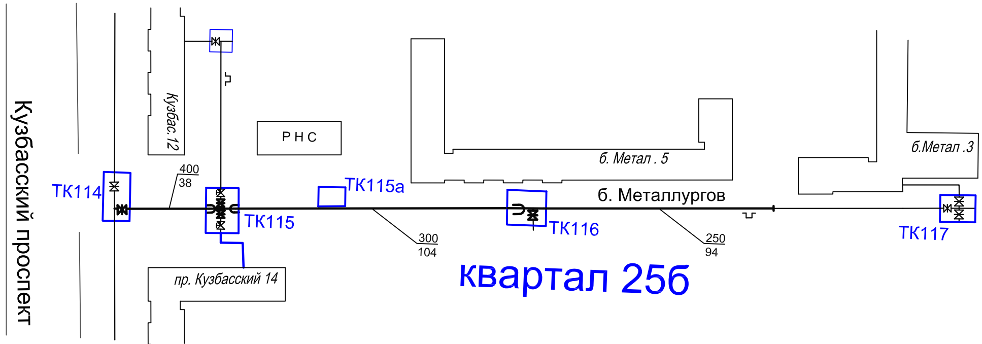
Схема квартальной тепловой сети
