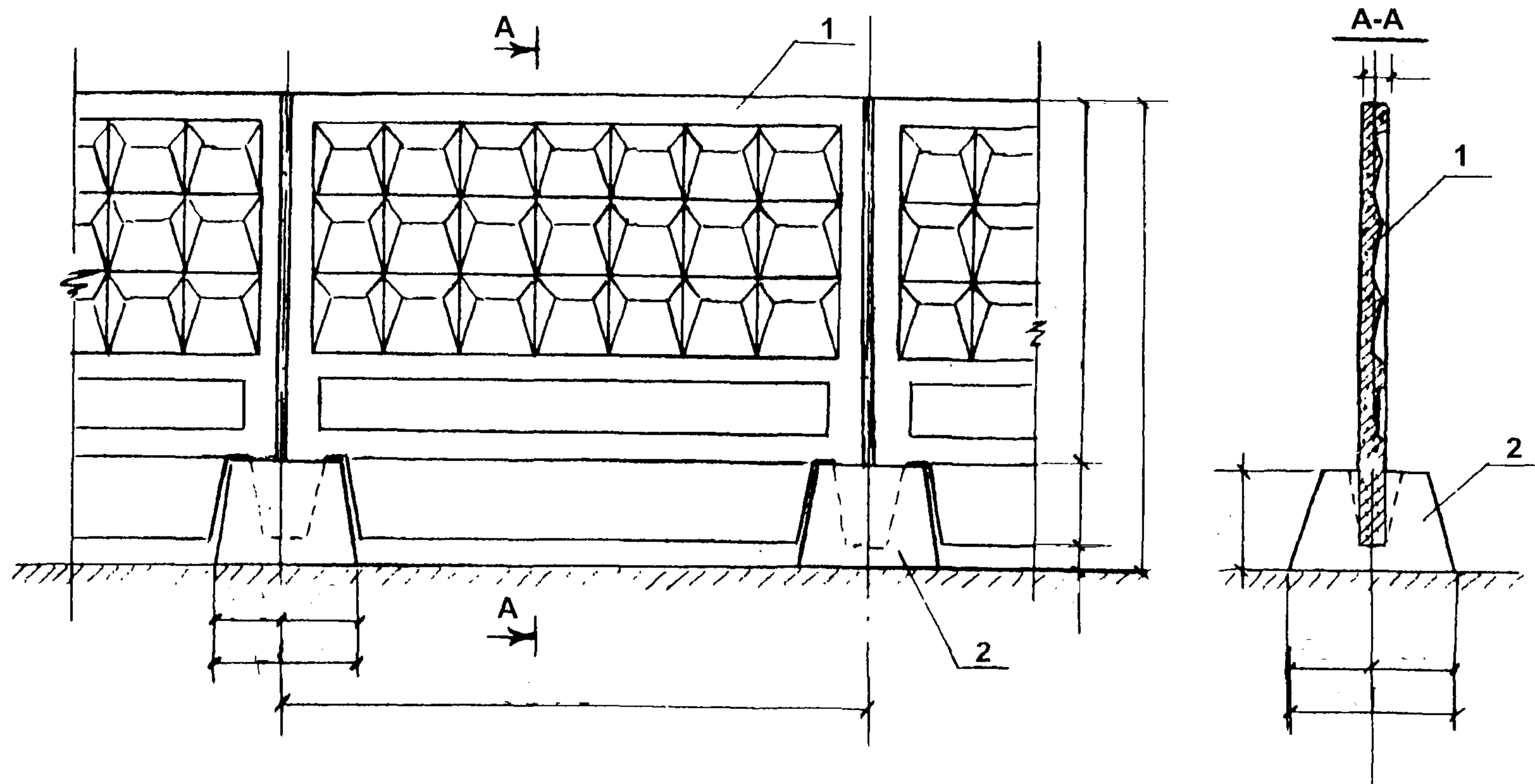
Рис. 6. Ограждение из сборных железобетонных элементов:
